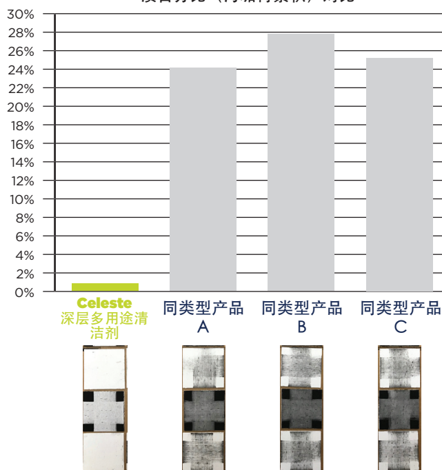
清洁期间重新沉积的ASTM A-6污渍百分比（污垢再累积）对比
